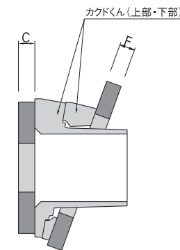
支圧板(アンカープレート)
