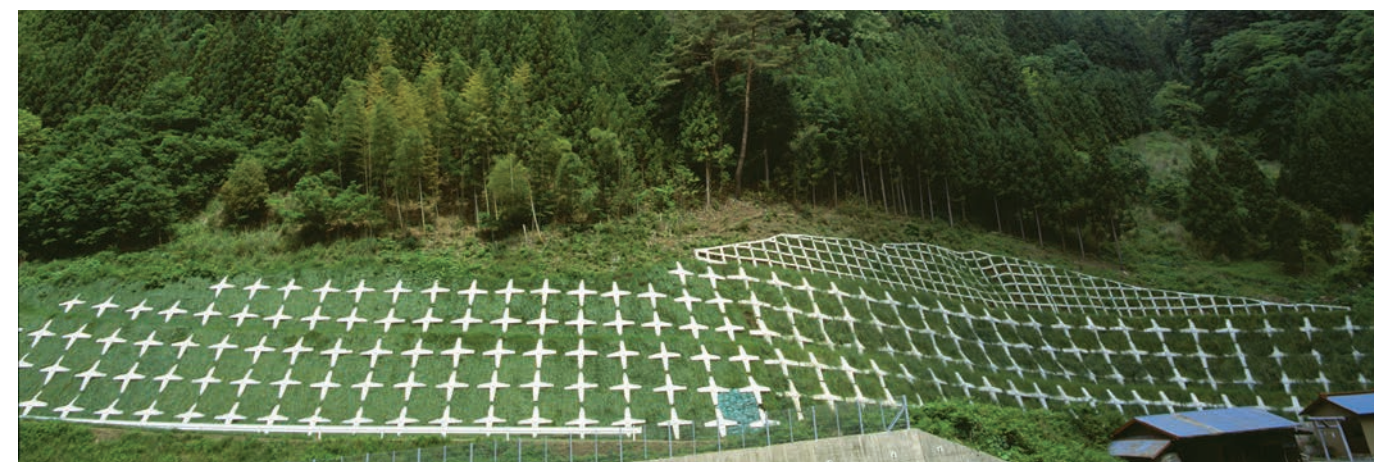
スーパーメタルフレーム(左) / PCフレーム(右) 三遠南信草木改良工事(静岡県)
