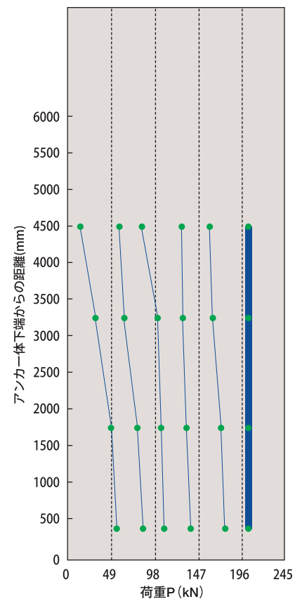
テンドン頭部変位から換算した荷重 全耐荷体
